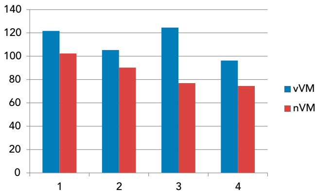
Abbildung 3: Variation der kapillaren Wasseraufnahme durch getrocknete Proben von Fichte, im Vergleich von Fälldaten in den 3.5 Tagen vor Vollmond (vVM) mit Fälldaten in den 3.5 Tagen nach Vollmond (nVM), für die Wintermonate November 2003 (1), Dezember (2), Januar 2004 (3) und Februar (4). Die Proben der «vor-Vollmond-Fälldaten» haben in den Monaten November, Dezember, Januar und Februar sehr deutlich mehr Wasser wieder aufgenommen als diejenigen der «nach-Vollmond-Daten».
