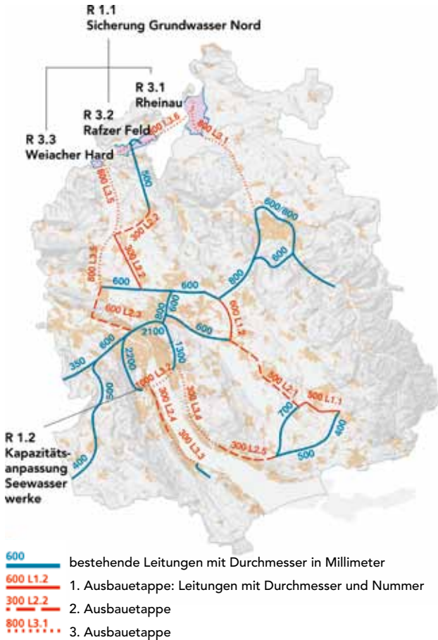
Abbildung 5: Leitungen des kantonalen Trinkwasserverbundes, Stand 2018
