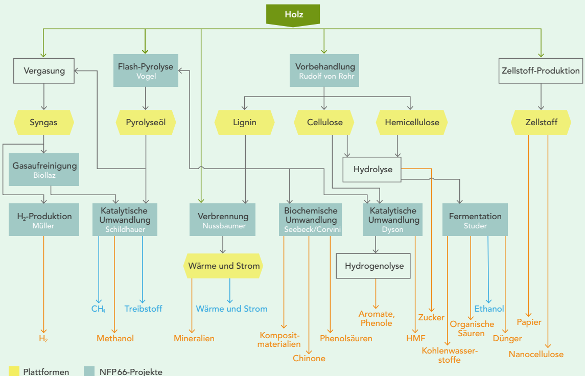
Abb. 1: Übersicht über Prozesse, Plattformen (Zwischenprodukte) und Endprodukte einer holzbasierten Bio Raffinerie (Cherubini et al., 2009; angepasst). Es sind hauptsächlich die Prozesse eingezeichnet, die im Rahmen des NFP 66 erforscht wurden. Die Namen der Projektleiter sind in weisser Schrift angegeben.
