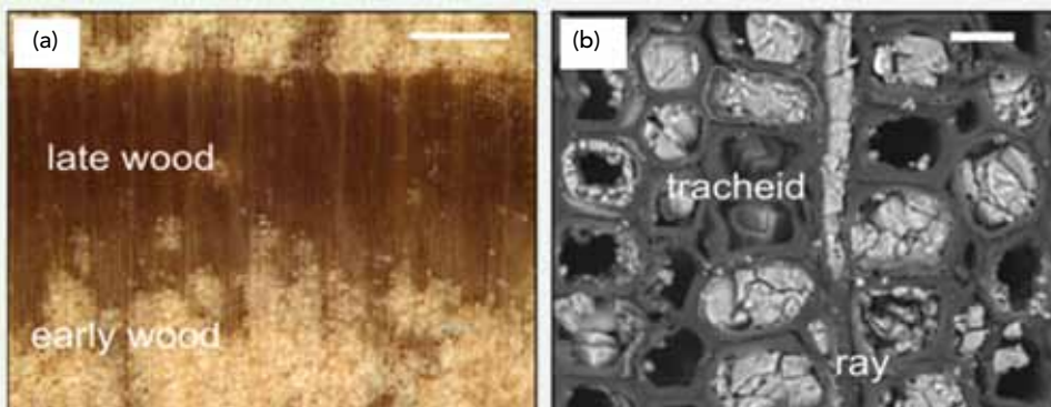
Abb. 1: Mineralisierte Fichte, (a) lichtmikroskopische Aufnahme, (b) rasterelektronenmikroskopische Aufnahme (Merk et al. 2016)
