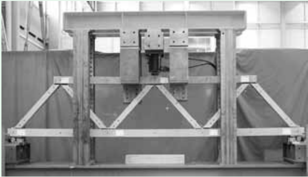
Abb. 4 : Duktiles Tragverhalten der entwickelten Fachwerke mit Furnierschichtholzplatten aus Buche
