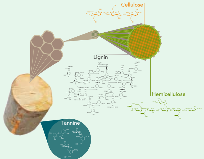
Abb. 2: Chemische Struktur von verholzter Biomasse. Die Zellwände von Holz bestehen aus Cellulose, Hemicellulose und Lignin. (angepasst von Neubauer, 2008).
